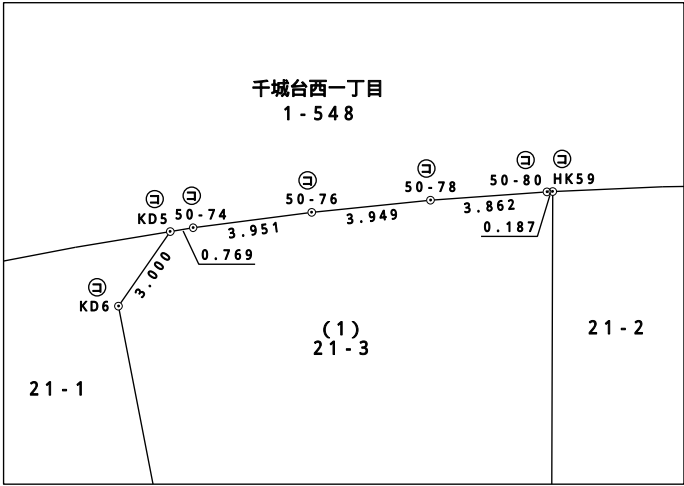
拡大図 S = 1 : 250
