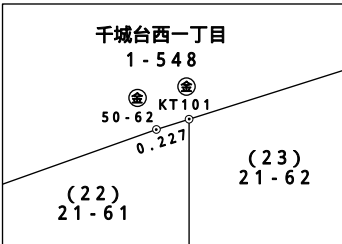
拡大図B S=1:50
