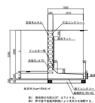
断面図 S=1:50
