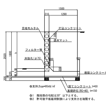
断面図 S=1:50
