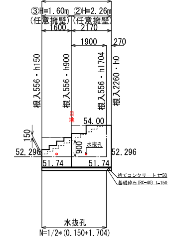
正面図 S=1:100 416-67区画・CP型枠擁壁（切土擁壁）
