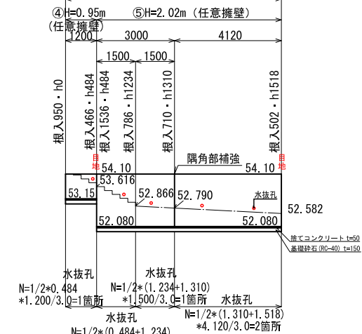
正面図 S=1:100 416-68区画・CP型枠擁壁（切土擁壁）
