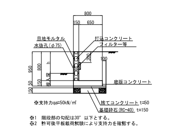
断面図 S=1:50
