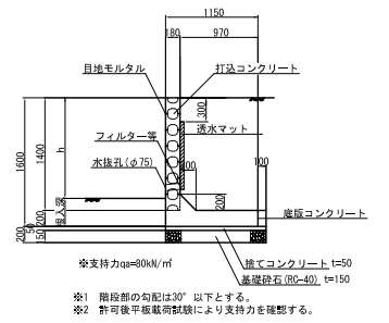
断面図 S=1:50
