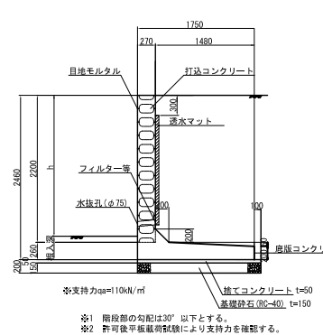
断面図 S=1:50
