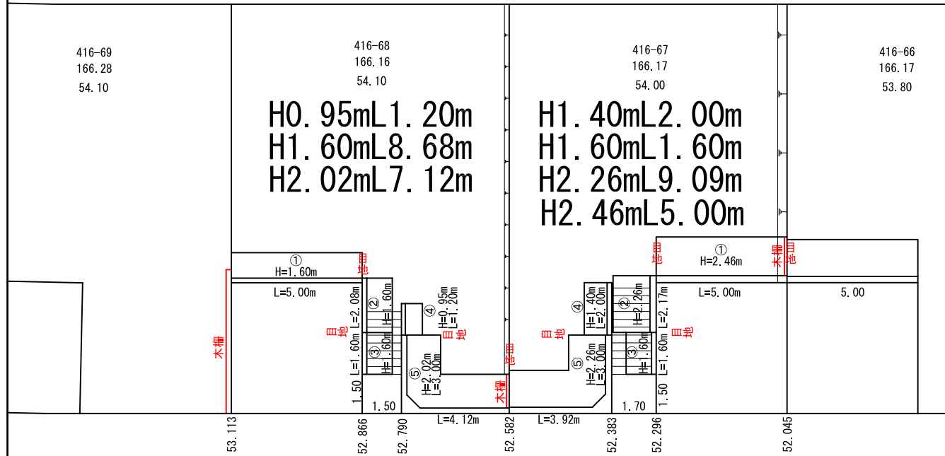
平面図 S=1:100
