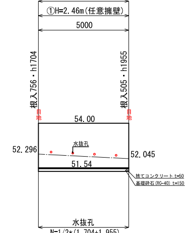
正面図 S=1:100 416-67区画・CP型枠擁壁（切土擁壁）
