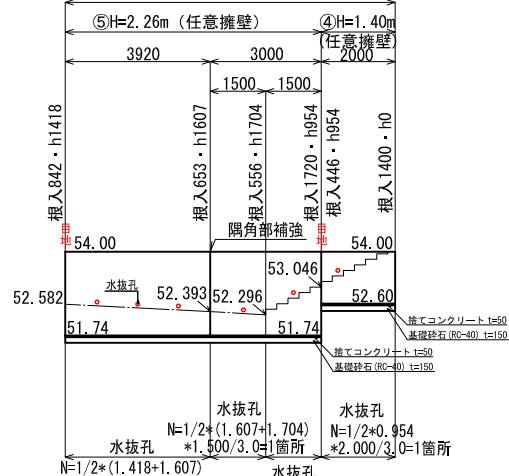
正面図 S=1:100 416-67区画・CP型枠擁壁（切土擁壁）
