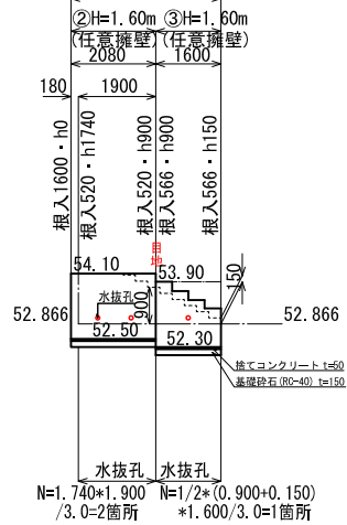
正面図 S=1:100 416-68区画・CP型枠擁壁（切土擁壁）
