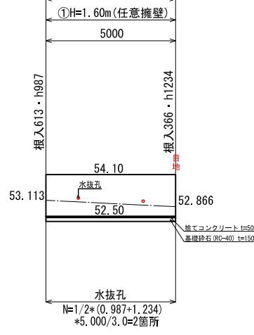
正面図 S=1:100 416-68区画・CP型枠擁壁（切土擁壁）
