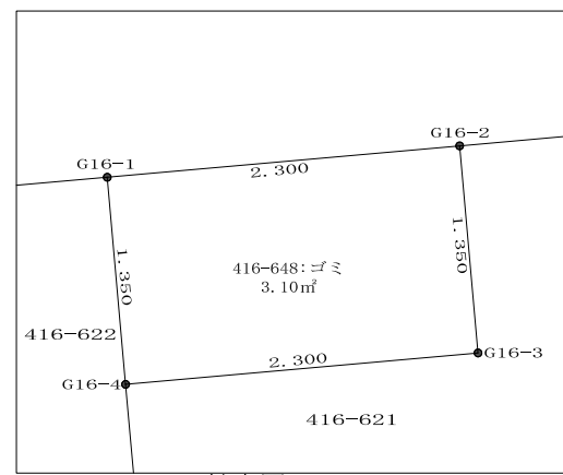
拡大図 S=1:50
